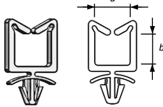
EK.27.1027 - EK.28.1028 - EK.30.1030
